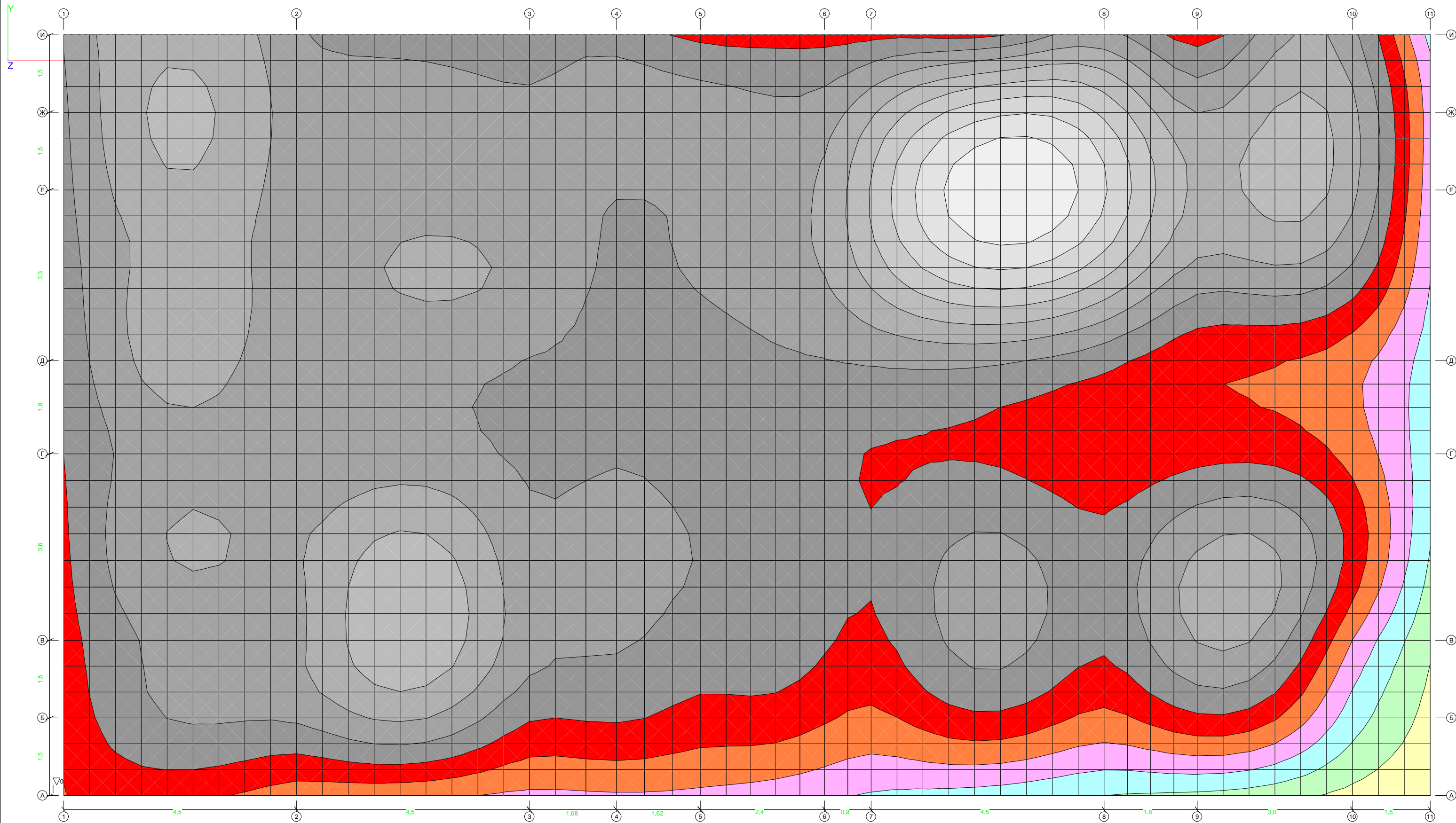
Перемещения Z (мм). Комбинация 1 ((L1)*1+(L2)*1+(L3)*1+(L4)*1+(L5)*1+(L6)*1+(L7)*1+(L16)*1)
