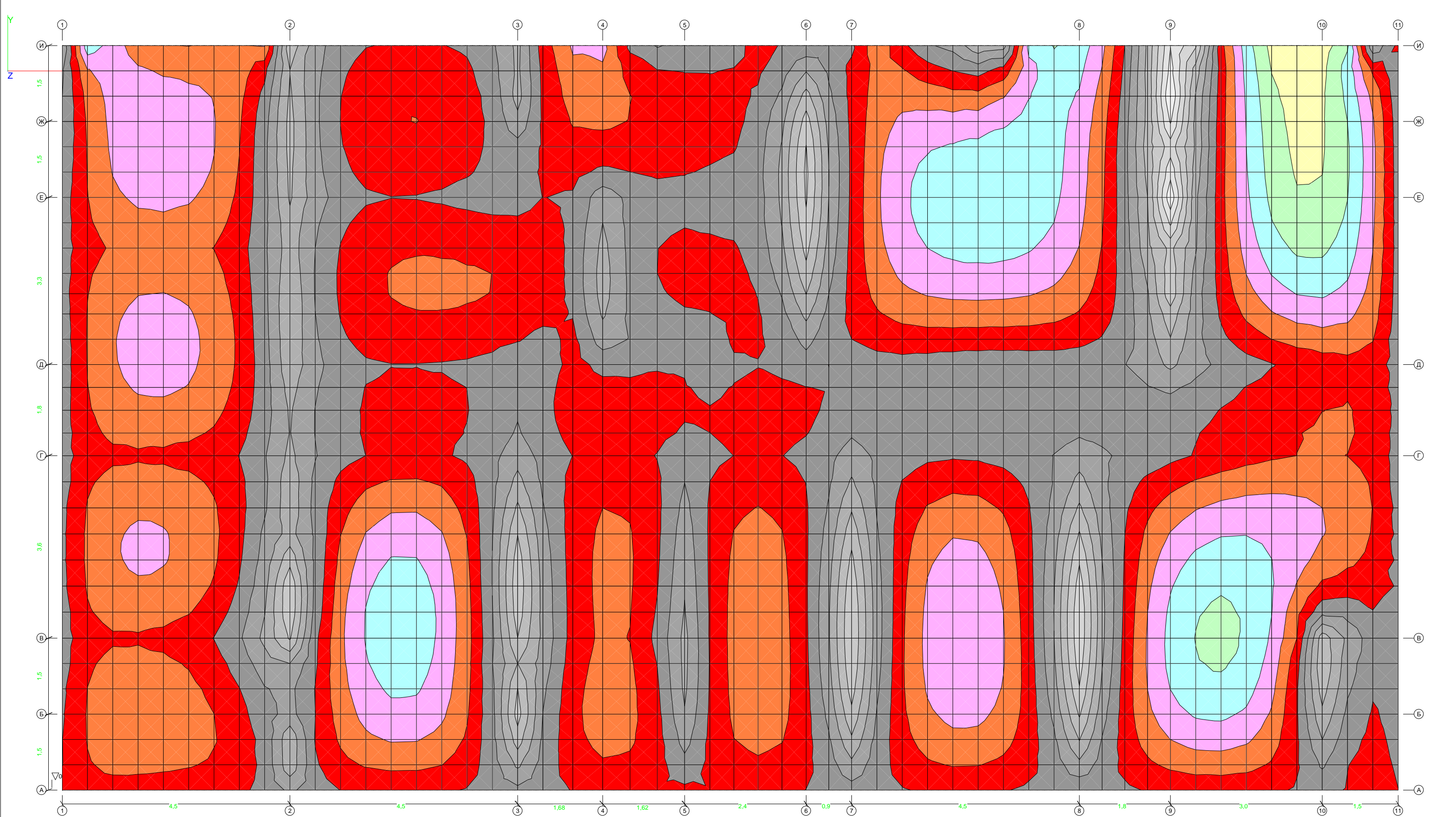
Корпус 13. Фундаментная плита. Моменты Мх
