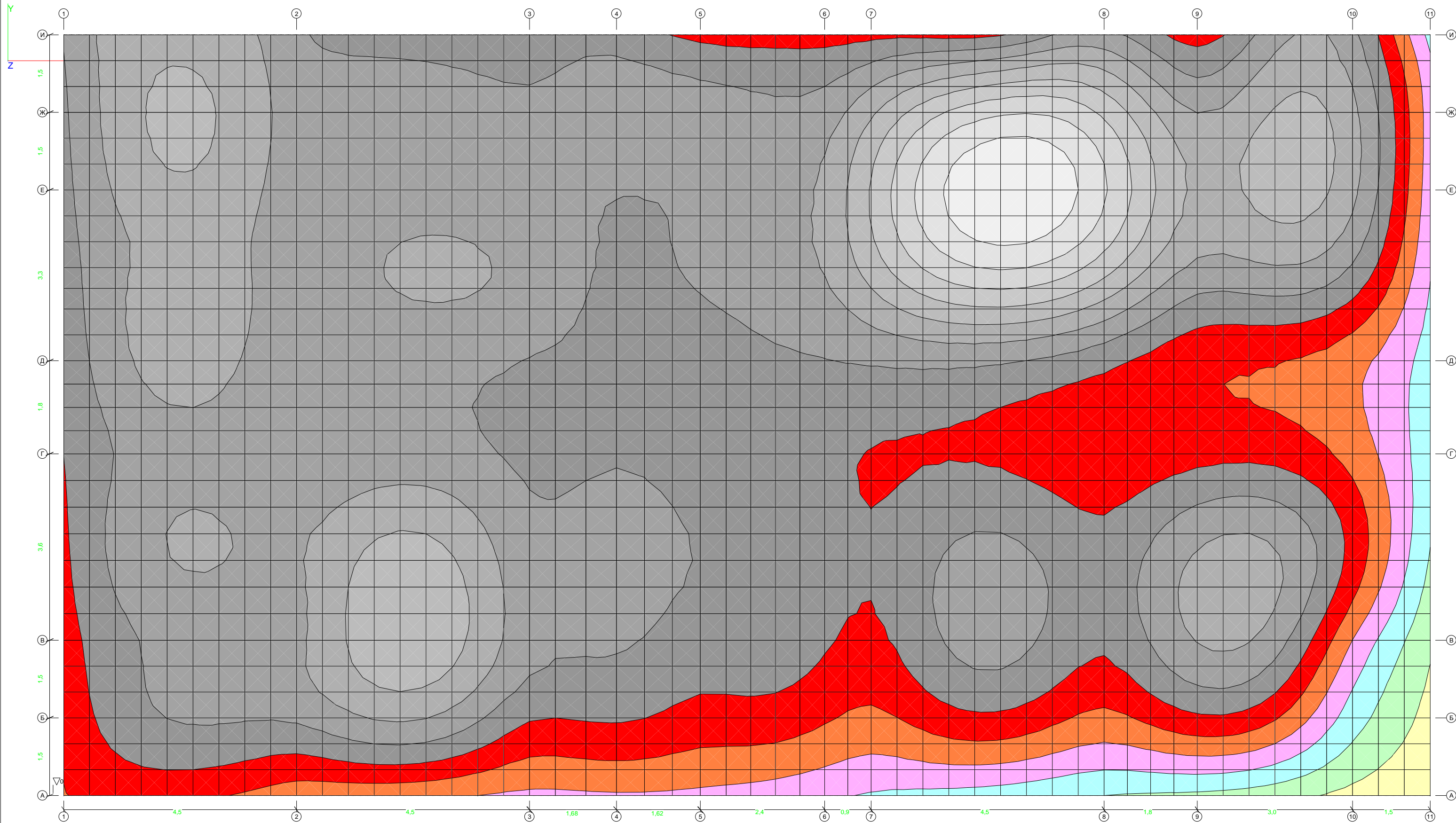
Корпус 13. Фундаментная плита. Отпор грунта Rz
