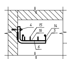
Разрез 2-2
