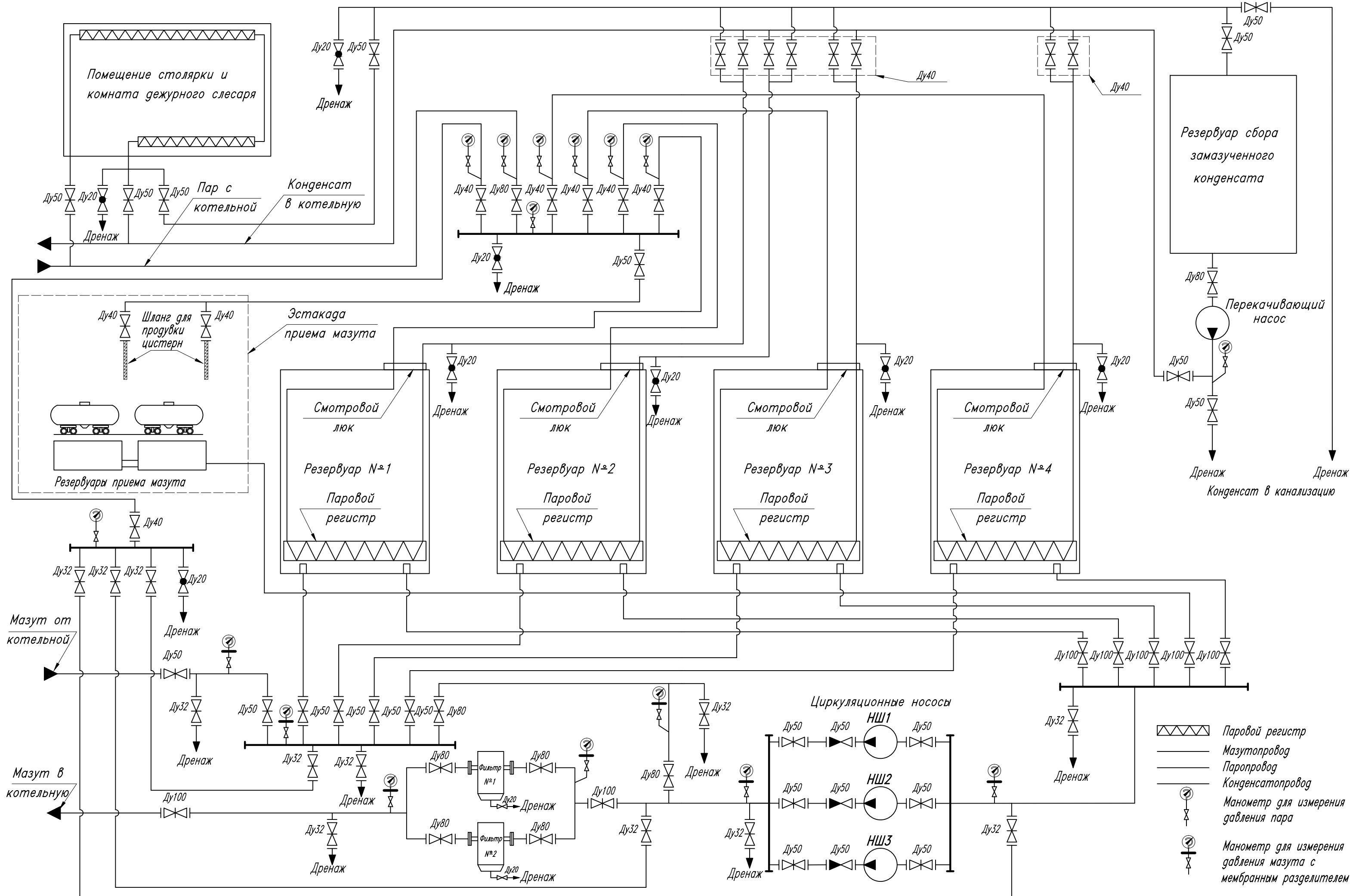
Технологическая схема реконструкции мазутонасосной станции
